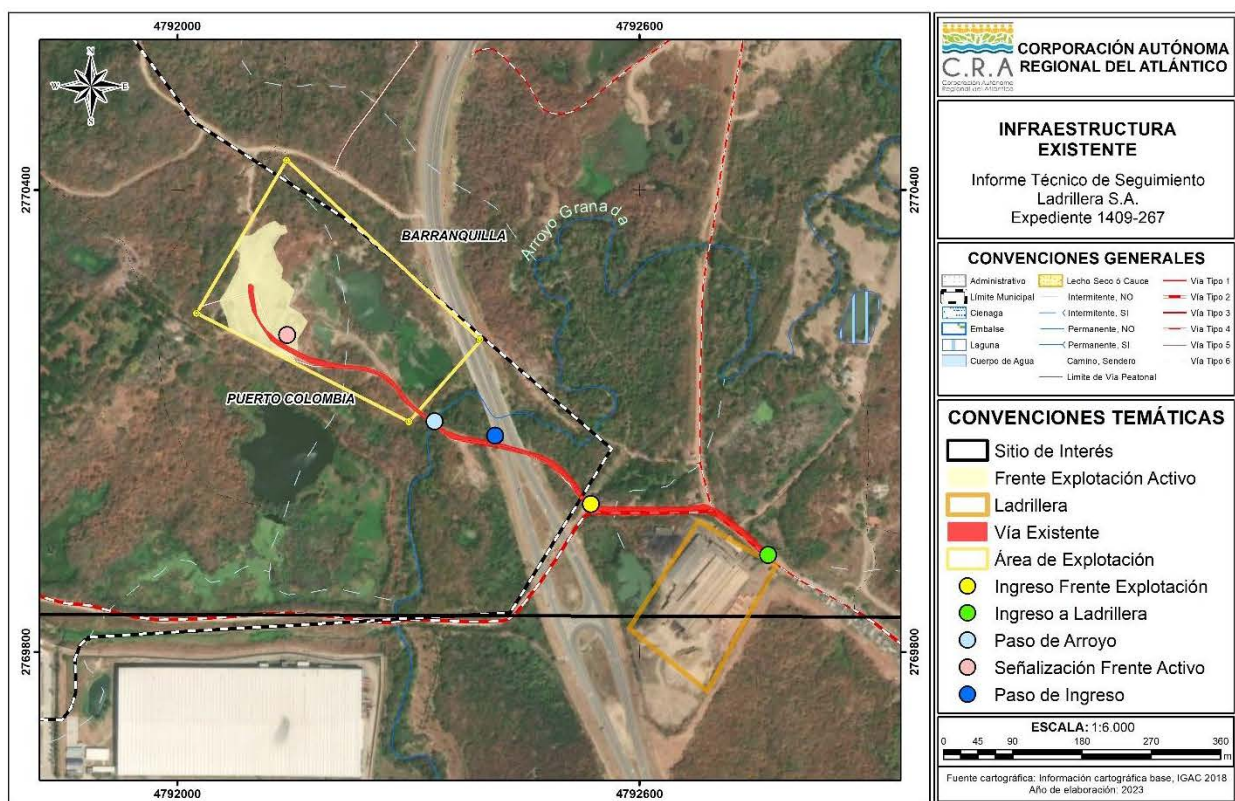
Figura 5. Infraestructura existente en el Título Minero 19812 y área licenciada de la Cantera denominada “El Bajo”.
